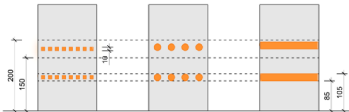
Rysunek 1 Sposoby oznakowania elementów transparentnych jak ściany i drzwi (Zał. nr 1 do MDS - rysunek nr 9) https://rarr.rzeszow.pl/projekty/projekt-dostepna-szkola/#dostepna-szkola-model-dostepnej-szkoly
